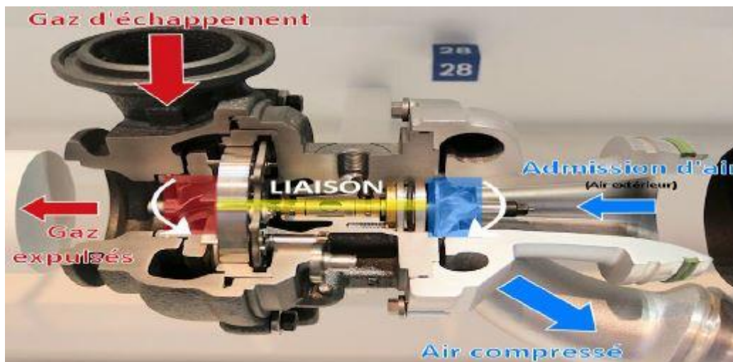
Figure I.5 : fonctionnement d'un turbocompresseur.
