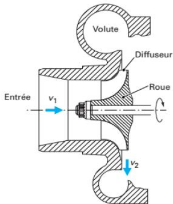
Figure 2 – Compresseur centrifuge : schéma
