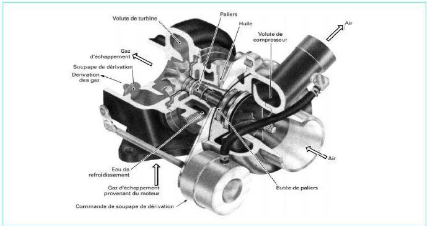
Figure 1 – Écorché de turbocompresseur d'automobile (source Garrett)
