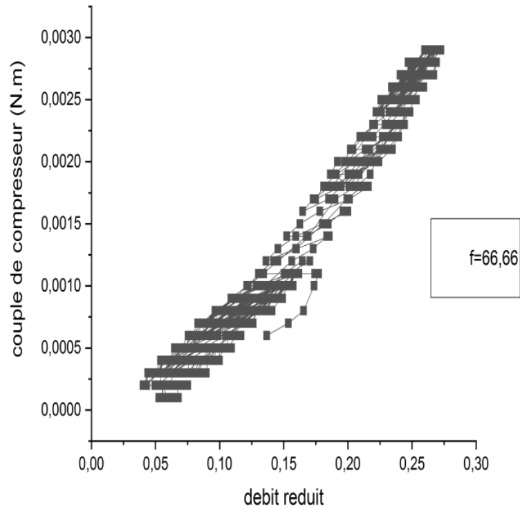
Figure III.10 : la variation de couple du compresseur en fonction de débite réduit
