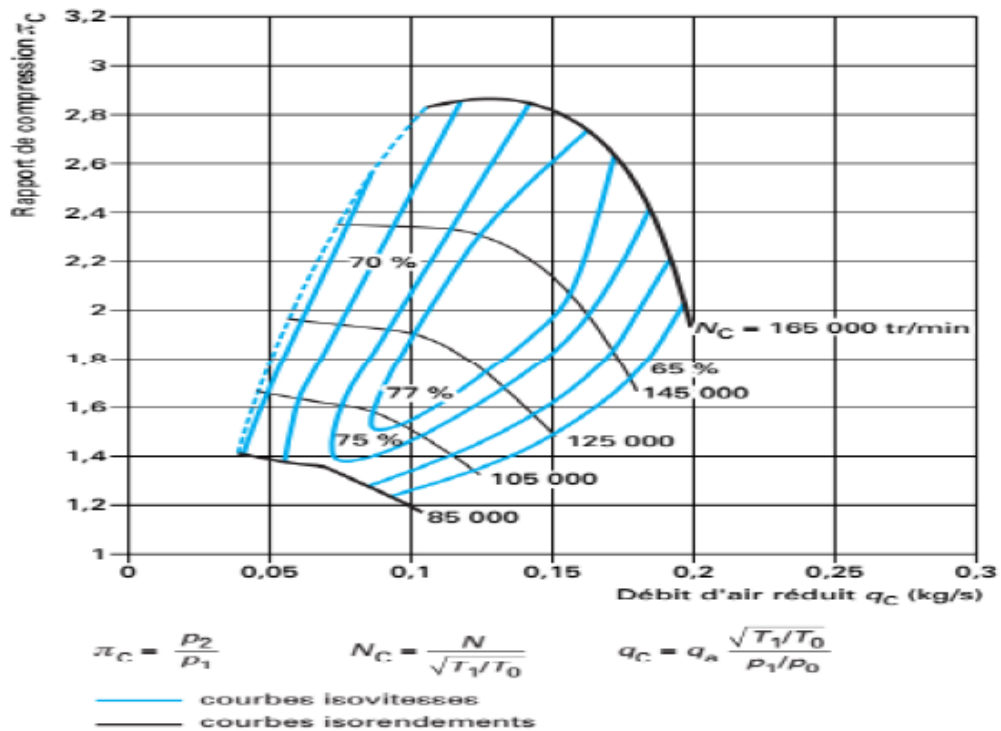
Figure 3– Caractéristique débit-pression d'un compresseur (champ compresseur) de moteur automobile (compresseur Garrett).
