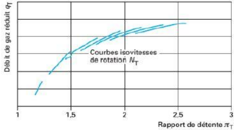
(a) courbes caractéristiques de débit
