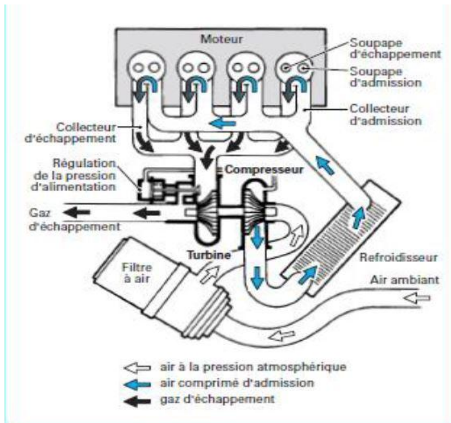
Figure I.2 : Installation d'un turbocompresseur sur un moteur automobile
