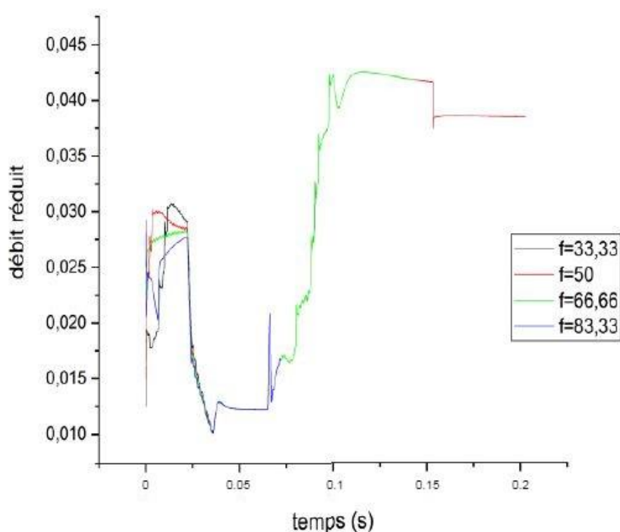
Figure III.2 : variation de débit réduit en fonction de temps (turbine).
