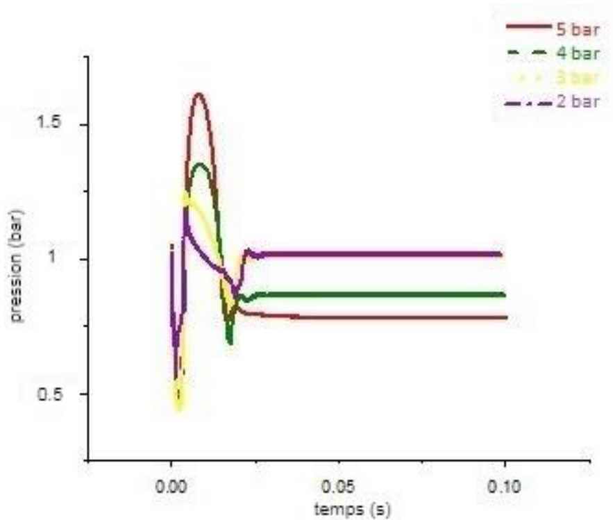
Figure III.9 : la variation de la pression en fonction du temps par différent pression
