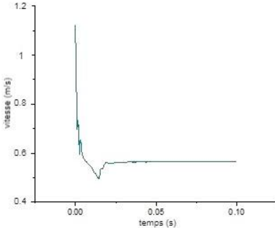
Figure III.8 : La variation de la vitesse du gaz d'échappement en fonction du temps
