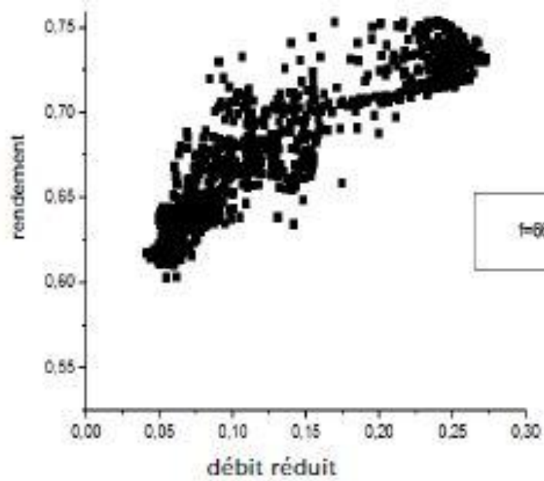
Figure III.14 : la variation de rendement de la turbine en fonction de débit réduit
