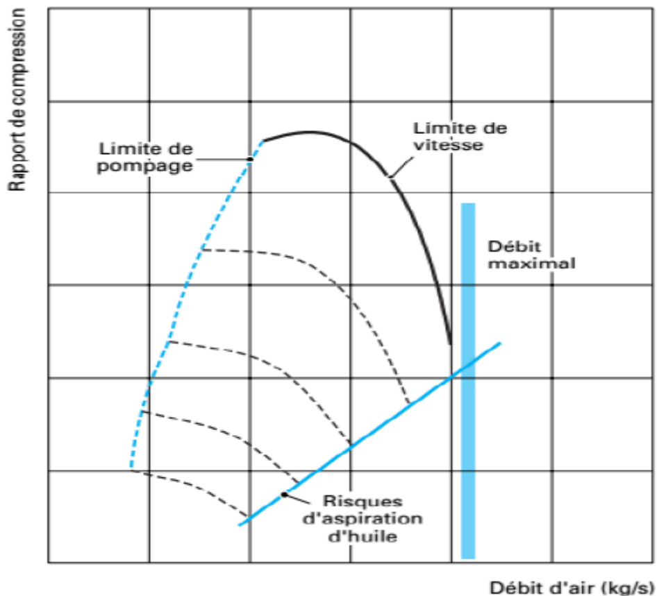
Figure 5 – Limites d'utilisation d'un compresseur
