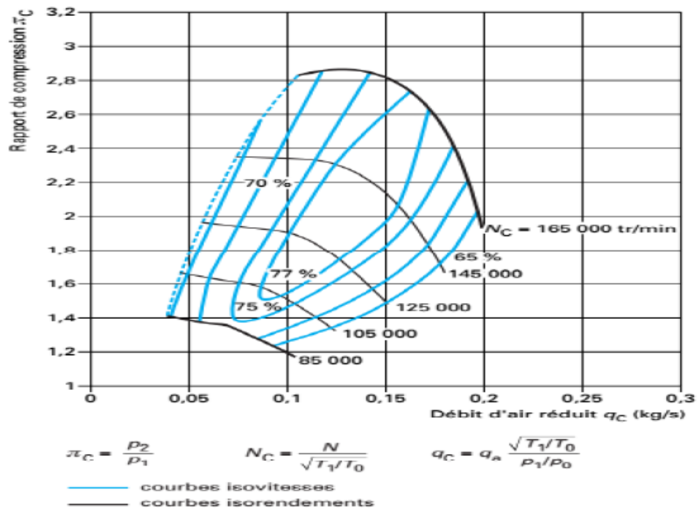
Figure 4– Caractéristique débit-pression d'un compresseur (champ compresseur) de moteur automobile (compresseur Garrett).
