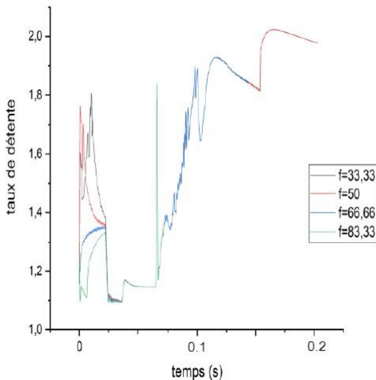
Figure III.3 : variation de taux de détente en fonction de temps (turbine).
