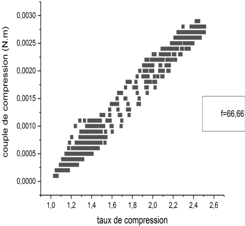
Figure III.12 : la variation de couple de la turbine en fonction de taux de compression
