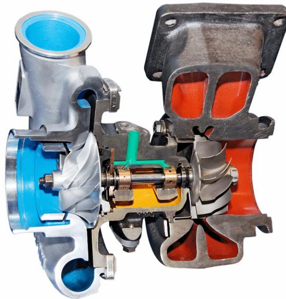
Figure I.3 : coupe d'un turbocompresseur
