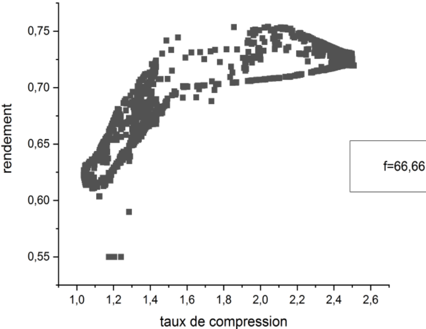
Figure III.13 : la variation de rendement de la turbine en fonction de taux de compression
