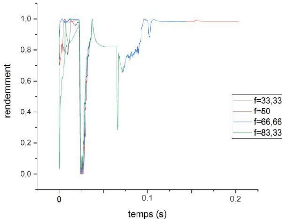
Figure III.4 : variation de rendement de la turbine en fonction de temps.
