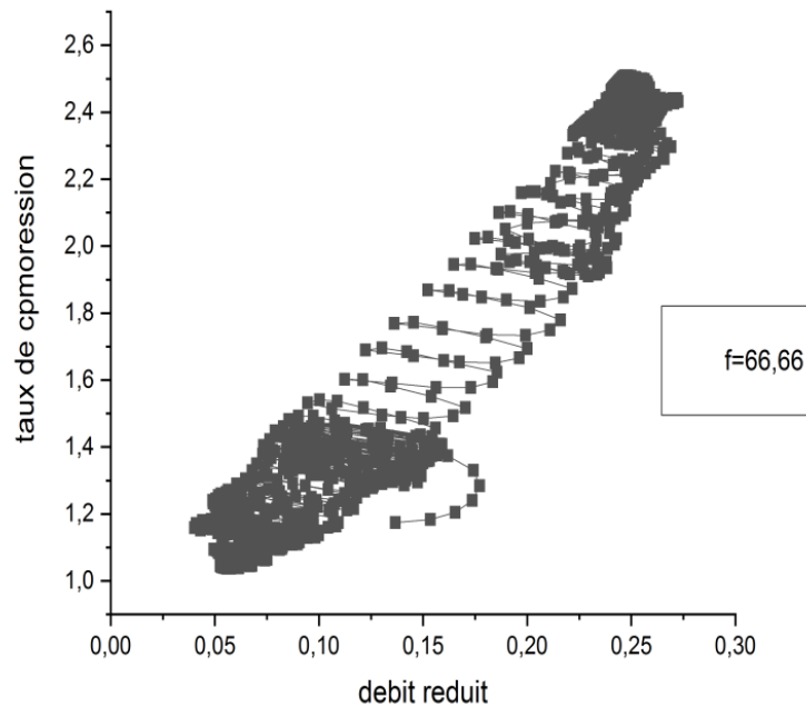
Figure III.11 : la variation de taux de détente en fonction de débite réduit
