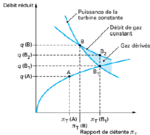
Figure 10 – Dérivation des gaz de turbine : caractéristique et points de fonctionnement.
