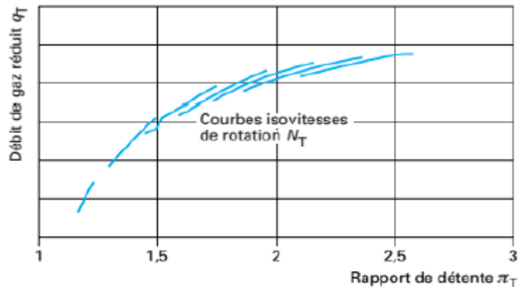
(a) courbes caractéristiques de débit
