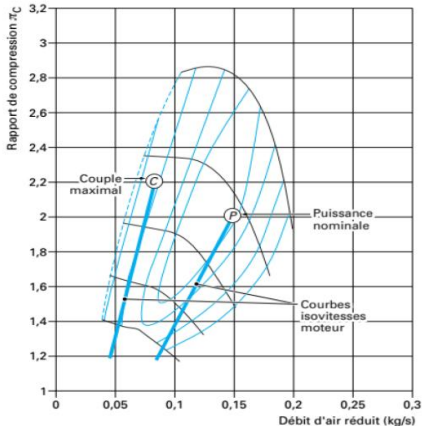
Figure 6 – Points de fonctionnement d'un compresseur.
