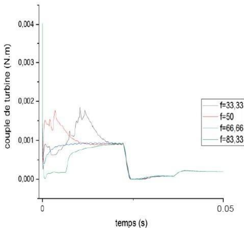
Figure III.5: variation de couple en fonction de temps (turbine).
