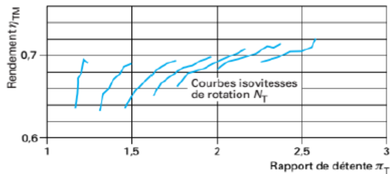
(b) courbes caractéristiques de rendement turbine-mécanique
