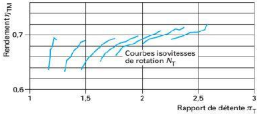
(b) courbes caractéristiques de rendement turbine-mécanique
