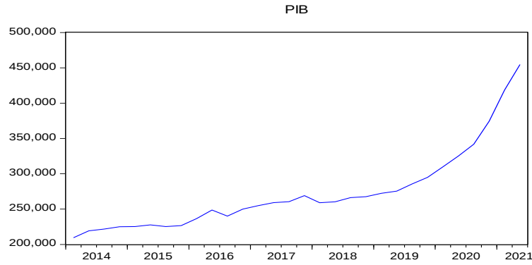
الشكل رقم 01: اتجاه عام لسلسلة زمنية (حالة اتجاه موجب)
