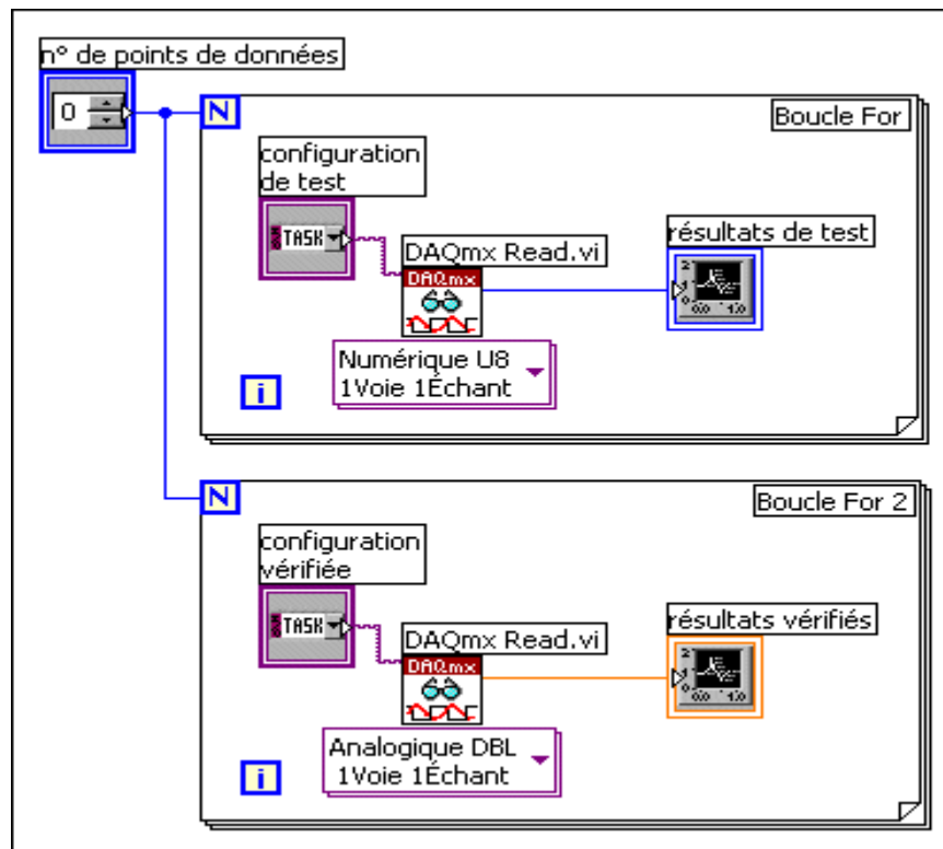
Figure. II.8: Exemple d'un flux de données à deux boucles "For" simultanées. [B9]
