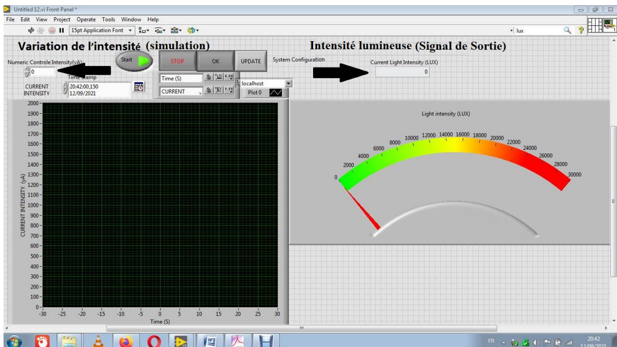
Figure III.10. Fenêtre du panneau avant sur LabVIEW qui affiche en temps réel les valeurs de la lumière mesurées en Lux.
