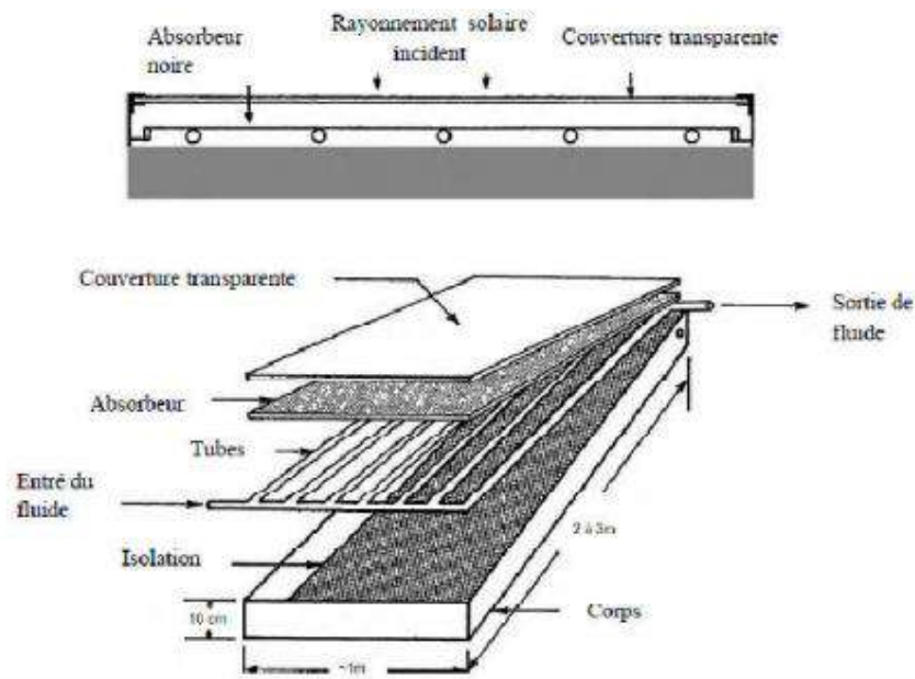
Figure I. 10: Vue en coupe d'un capteur plan. [16]
