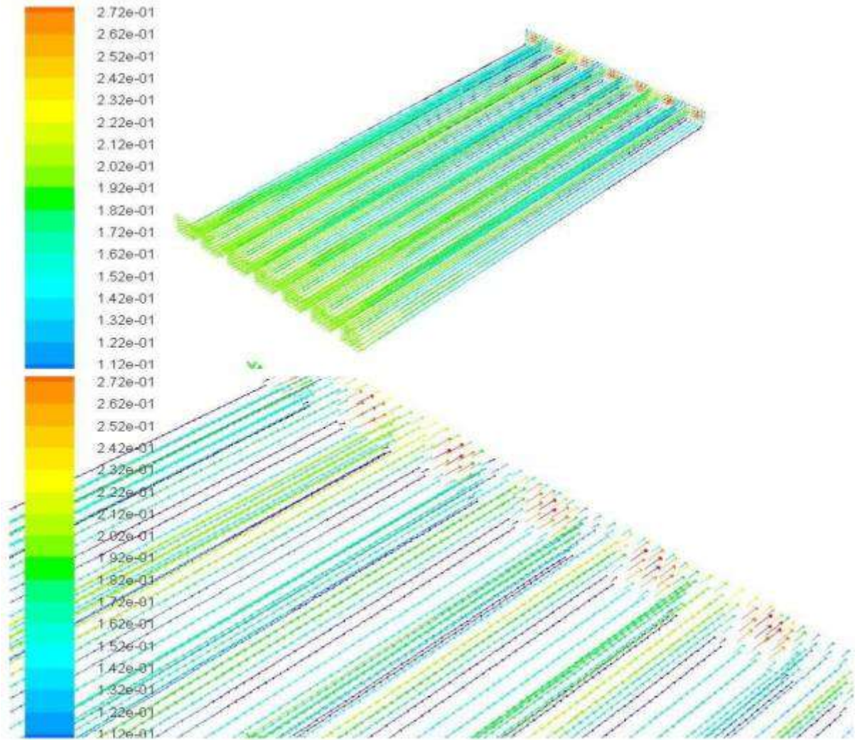
Figure IV. 5: Champ de vecteur de vitesse pour différentes hauteur d'ailettes de capteur à une intensité solaire de 618 \text{ W/m}^2 .
