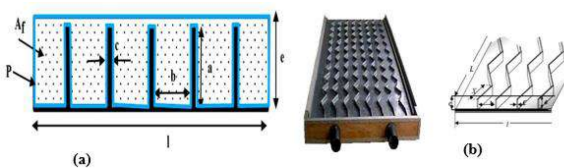
Figure II. 12: (a) Vue en coupe droite d'une rangée de chicanes longitudinales et (b) Caractéristiques géométriques de chicanes longitudinales. [36]
