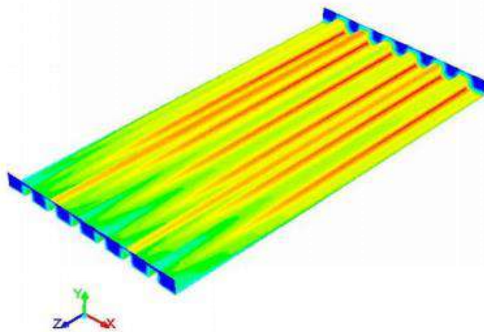
Figure IV. 4: Contours de la température pour différentes hauteurs d’ailettes à une intensité solaire de 618 \text{ W/m}^2 .
